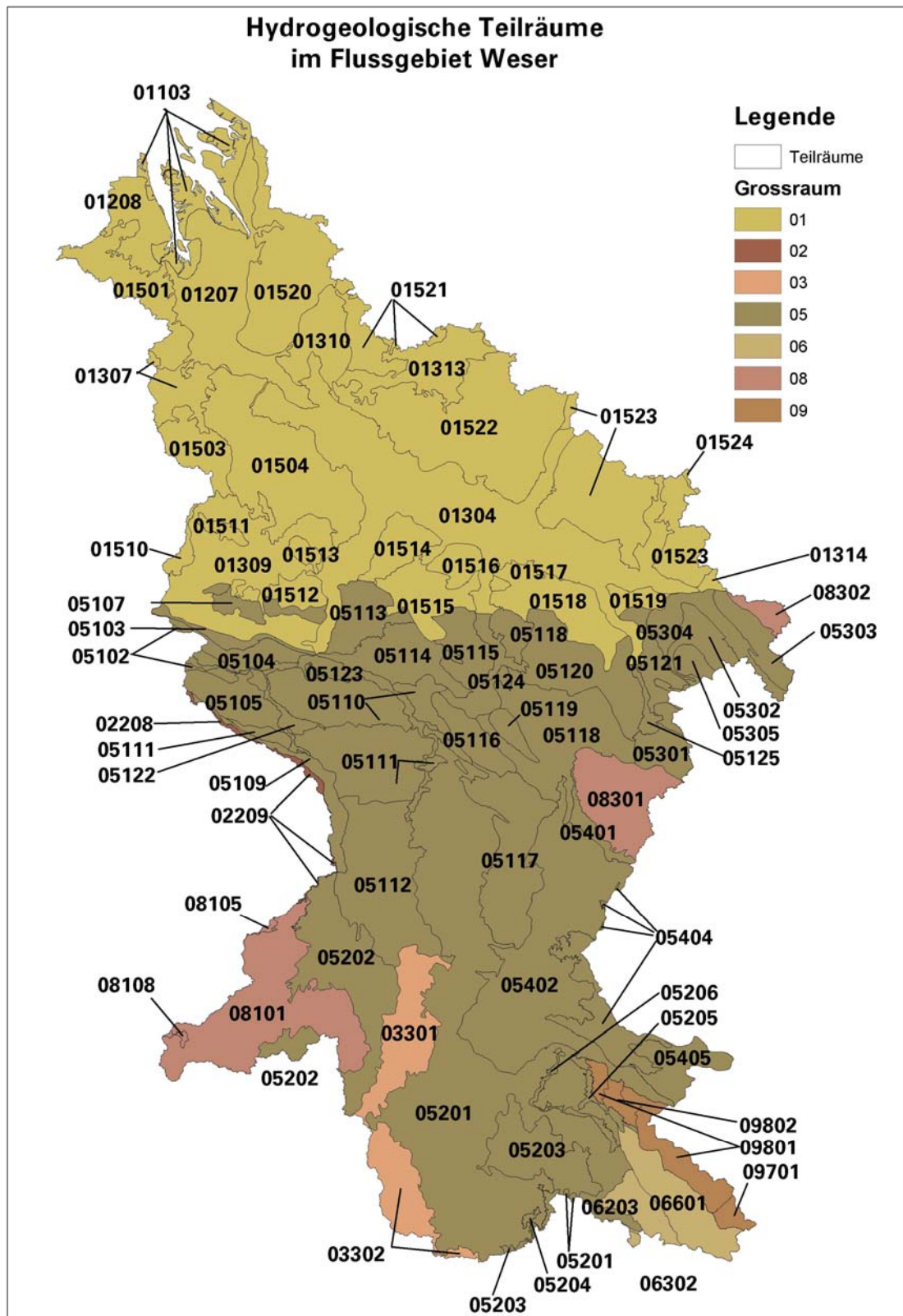
Hydrogeologische Teilräume im Flussgebiet Weser
